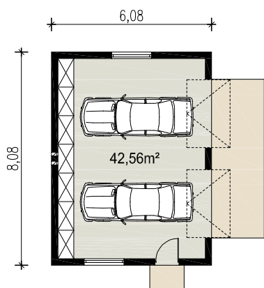
RZUT PARTERU
